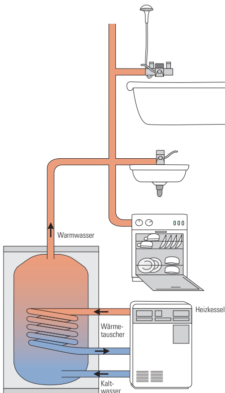
Warmwasserbereitung im Speichersystem mit indirekter Beheizung
