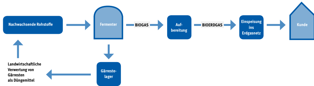
Schematische Darstellung einer Biogasanlage vom Einsatzstoff zum Haushaltskunden
